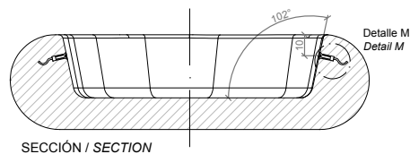
SECCIÓN / SECTION
