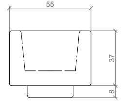
PERFIL / PROFILE
