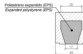
SECCIÓN B-B' / SECTION B-B'
