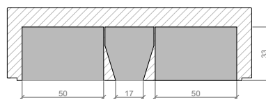
SECCIÓN A-A' / SECTION A-A'
